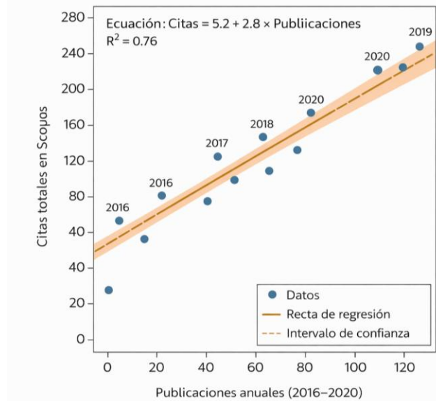
Gráfico 2. Recta de regresión.
