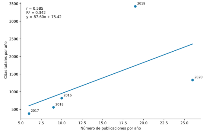
Gráfica 1. Dispersión publicaciones vs citas.
