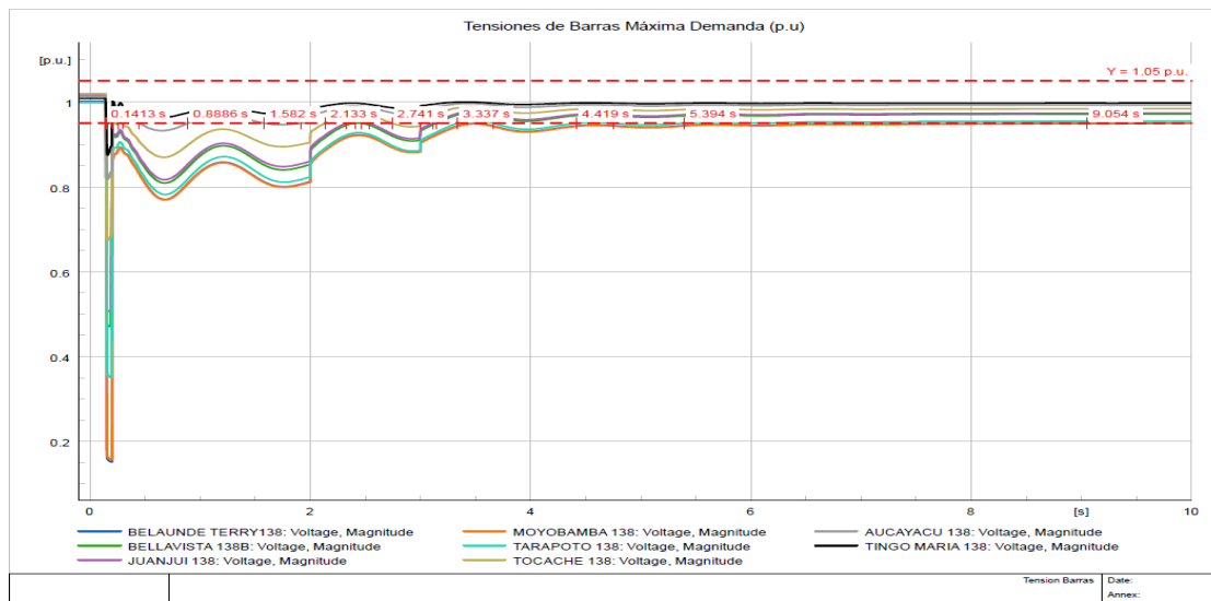
Figura 6: Valores de tensión en contingencia 2 aplicando propuesta de porcentajes de rechazo automático de carga en escenario a máxima demanda.
