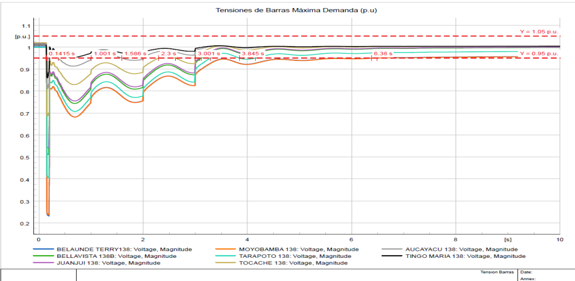
Figura 5: Valores de tensión en contingencia 1, maplicando propuesta de porcentajes de rechazo automático de carga en escenario a máxima demanda.
