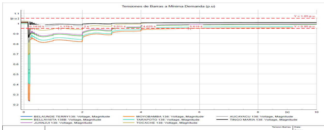
Figura 7: Valores de tensión en contingencia 1 aplicando propuesta de porcentajes de rechazo automático de carga en escenario a mínima demanda.
